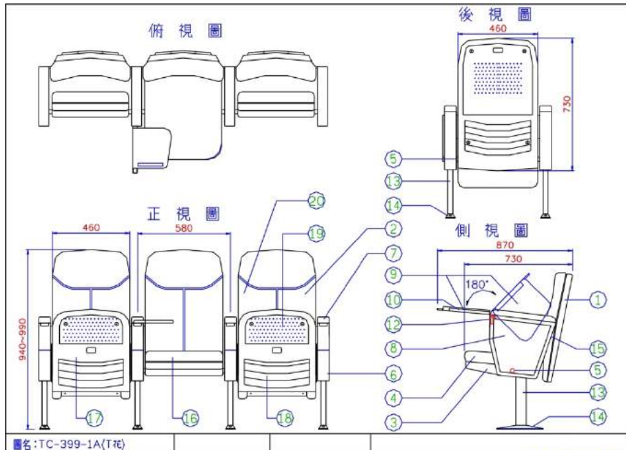
圖名: TC-399-1A(T花)
