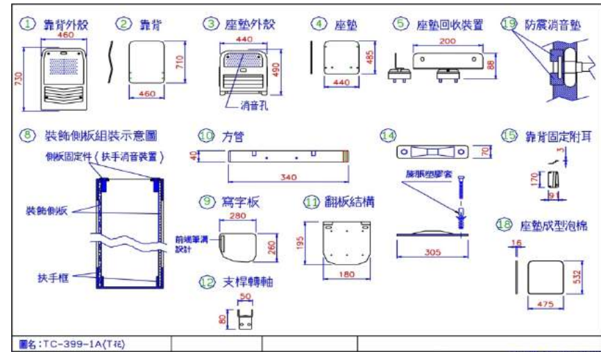
圖名: TC-399-1A(T花)
